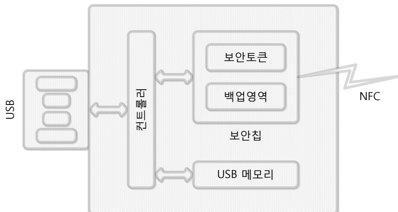
그림 2. KeyToken USB의 구성도
